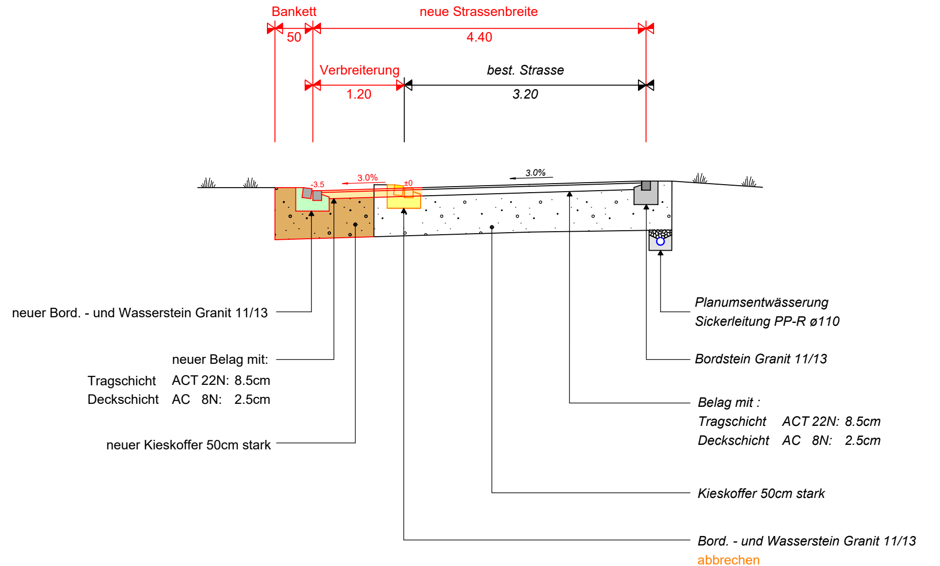
Profil 2 1:50 (Normalprofil)
