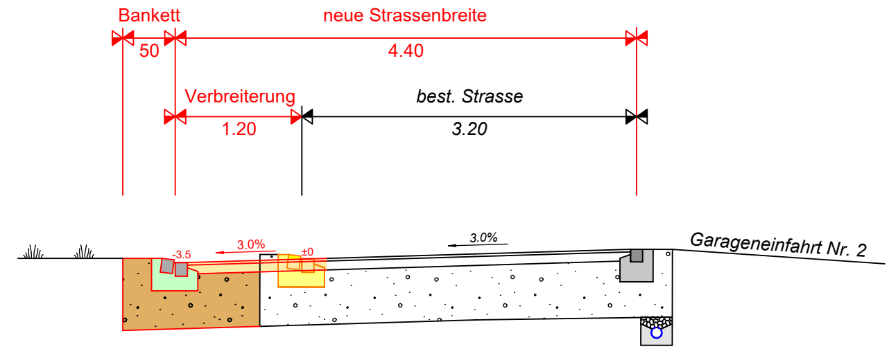
Profil 1 1:50
